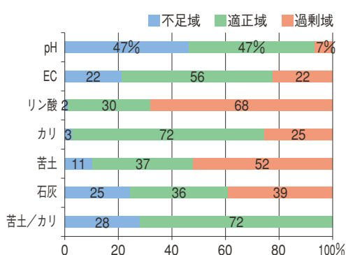
図－1 診断基準値に基づく施設土壌養分の状態
